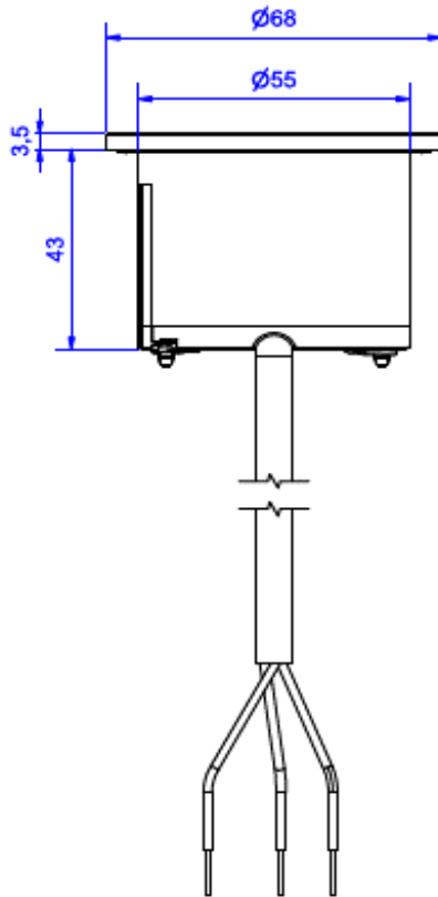
Montagestecker 31M
